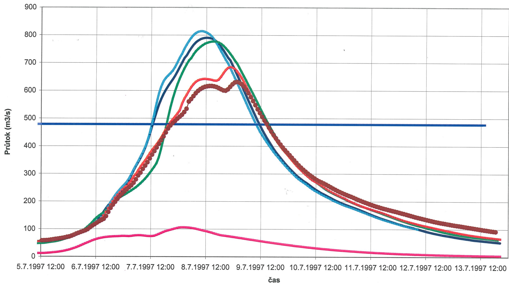
Povodeň v profilu pod Třebůvkou vyvolaná 100% srážkových úhrnů povodně 1997 v povodí
