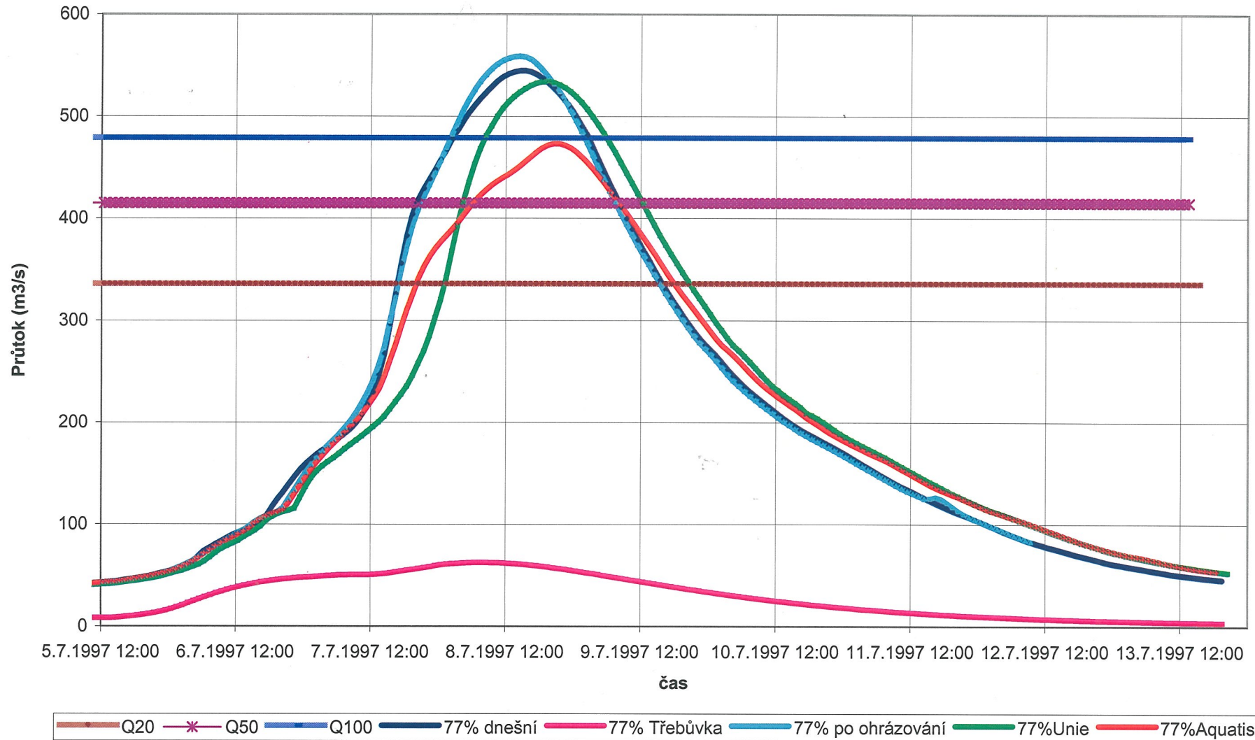
Povodeň v profilu pod Třebůvkou vyvolaná 77% srážkových úhrnů povodně 1997 v povodí
