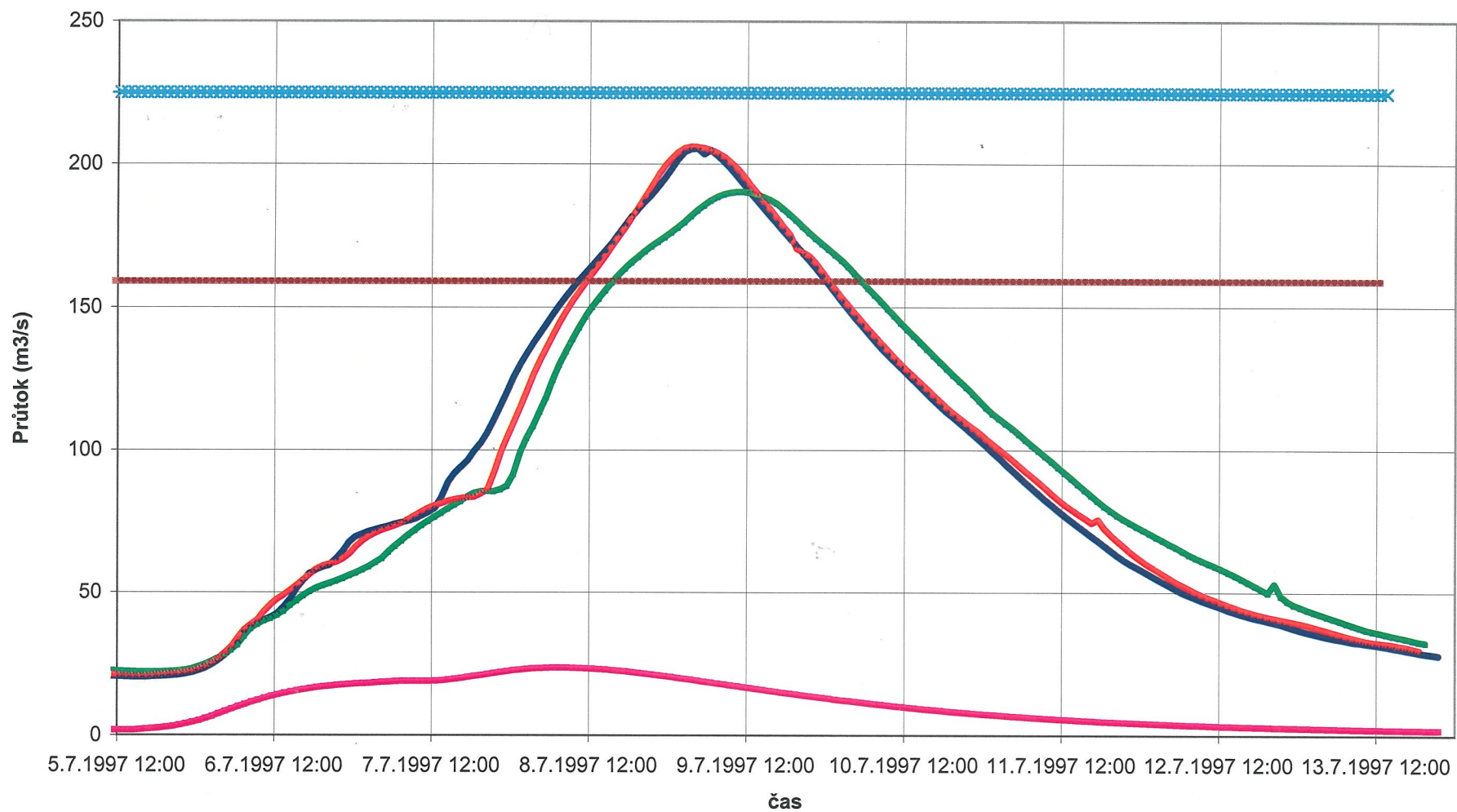
Povodeň v profilu pod Třebůvkou vyvolaná 40% srážkových úhrnů povodně 1997 v povodí
