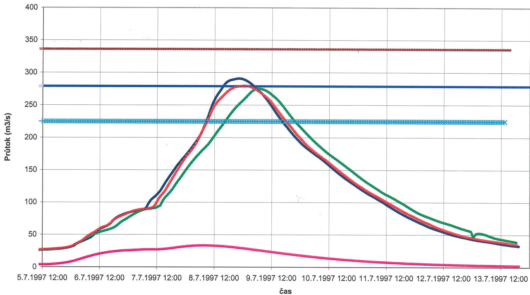
Povodeň v profilu pod Třebůvkou vyvolaná 50% srážkových úhrnů povodně 1997 v povodí
