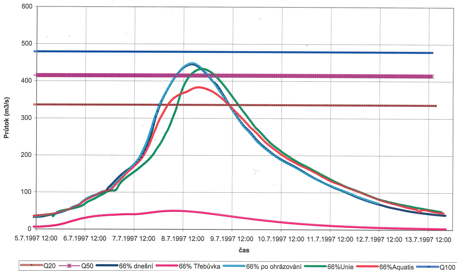
Povodeň v profilu pod Třebůvkou vyvolaná 66% srážkových úhrnů povodně 1997 v povodí
