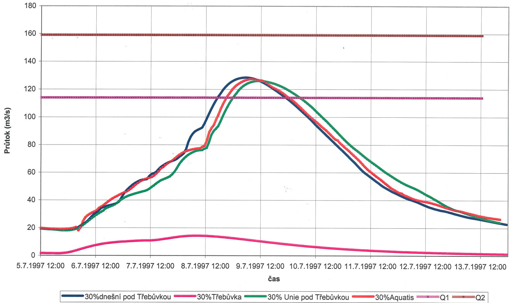
Povodeň v profilu pod Třebůvkou vyvolaná 30% srážkových úhrnů povodně 1997
