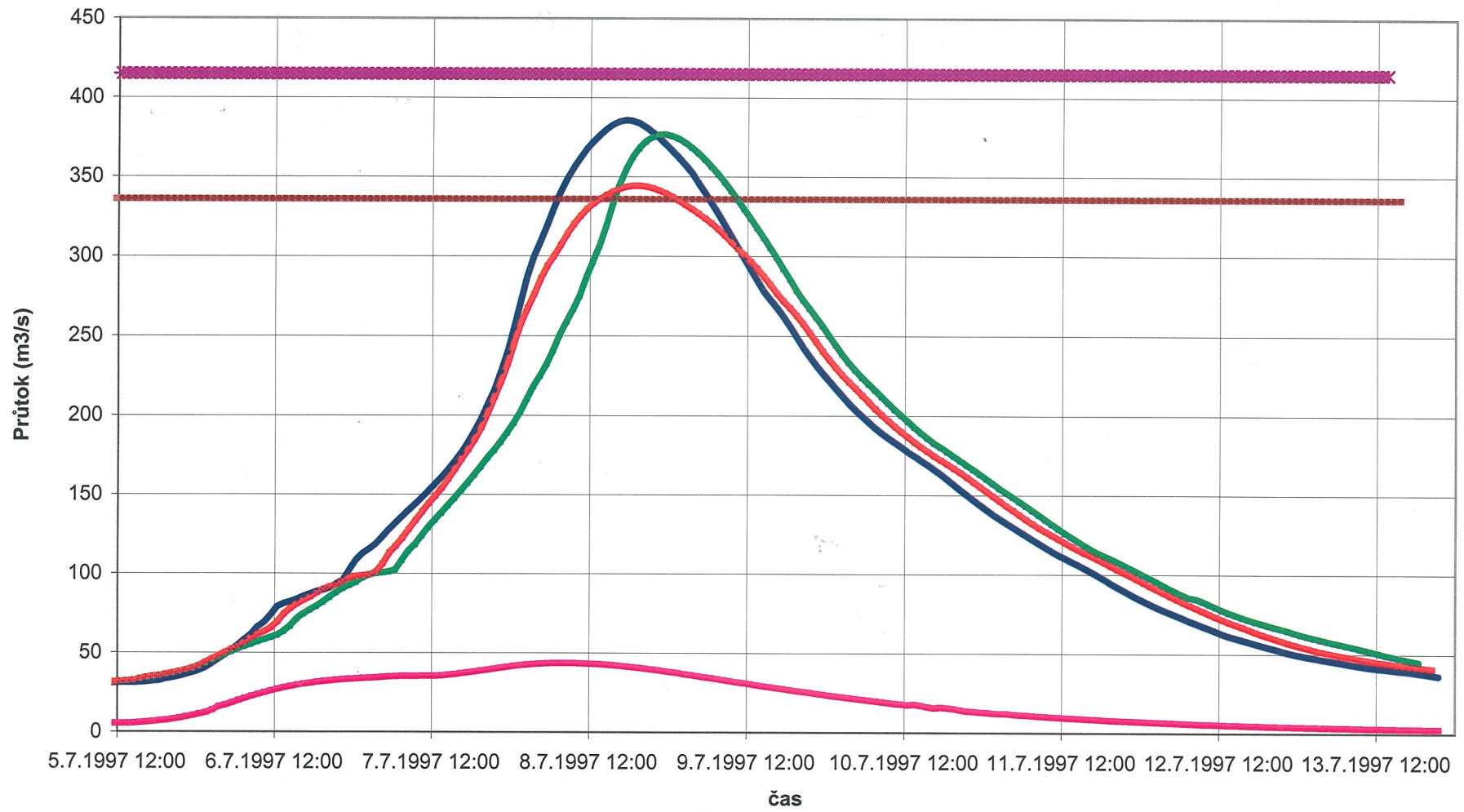
Povodeň v profilu pod Třebůvkou vyvolaná 60% srážkových úhrnů povodně 1997 v povodí
