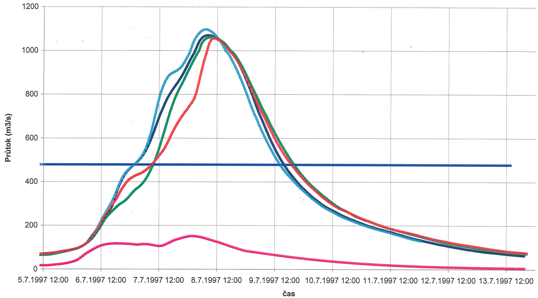
Povodeň v profilu pod Třebůvkou vyvolaná 125% srážkových úhrnů povodně 1997 v povodí
