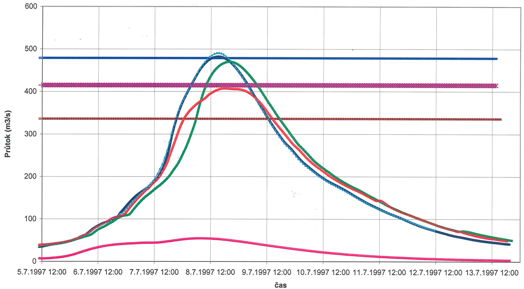
Povodeň v profilu pod Třebůvkou vyvolaná 70% srážkových úhrnů povodně 1997 v povodí
