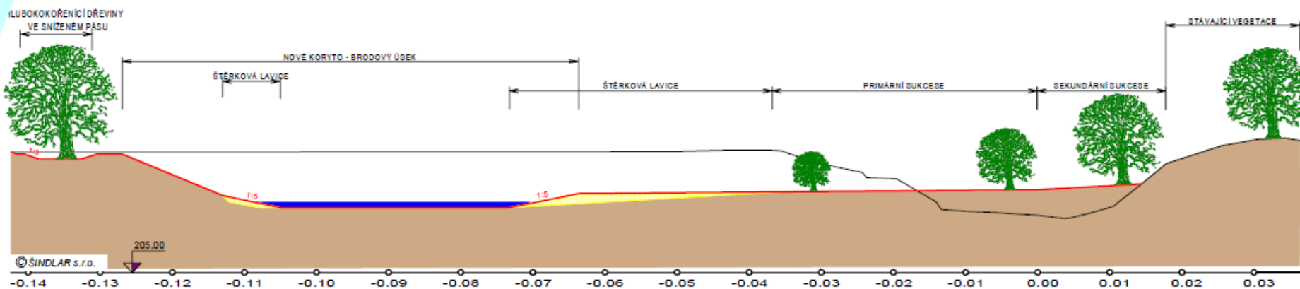
VZOROVÝ PŘÍČNÝ ŘEZ 2
