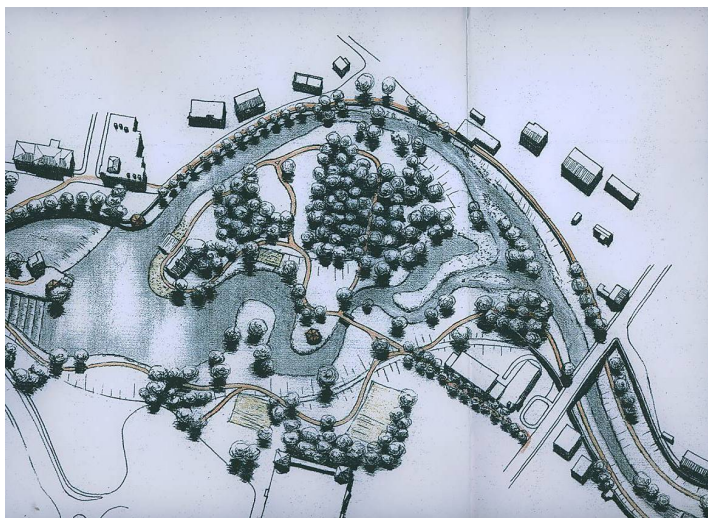
Obr. 4 Ukázka z navrhovaného řešení zvětšení kapacity koryta řeky Opavy a jejího zapojení do konceptu městské zeleně v Krnově
