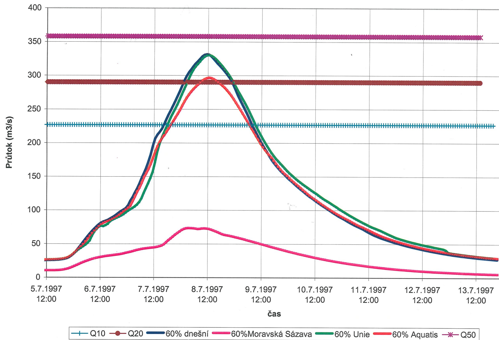
Povodeň v profilu pod Moravskou Sázavou vyvolaná 60% srážkových úhrnů povodně 1997
