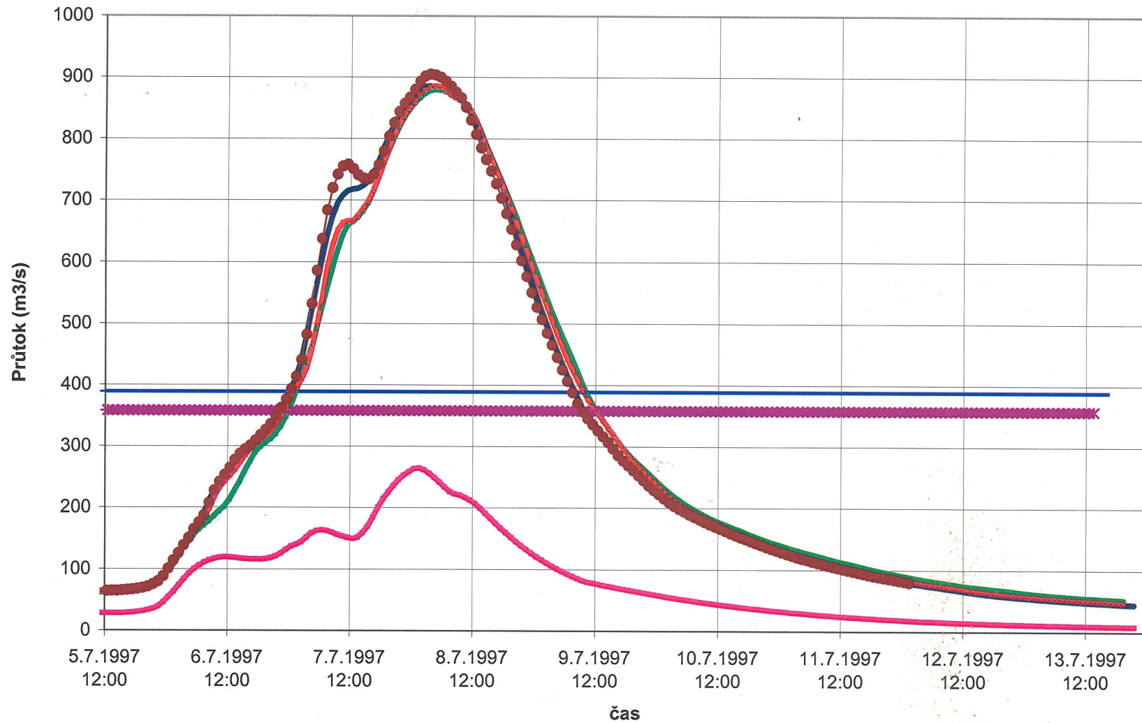
Povodeň v profilu pod Moravskou Sázavou vyvolaná 125% srážkových úhrnů povodně 1997
