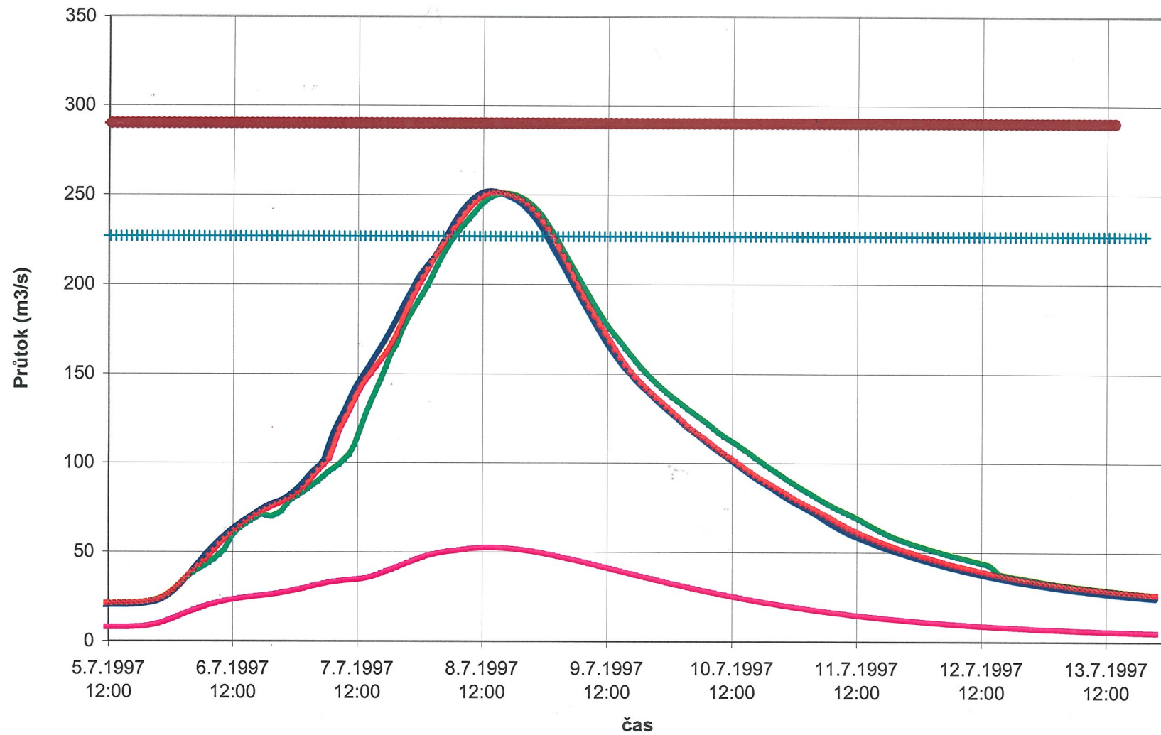
Povodeň v profilu pod Moravskou Sázavou vyvolaná 50% srážkových úhrnů povodně 1997
