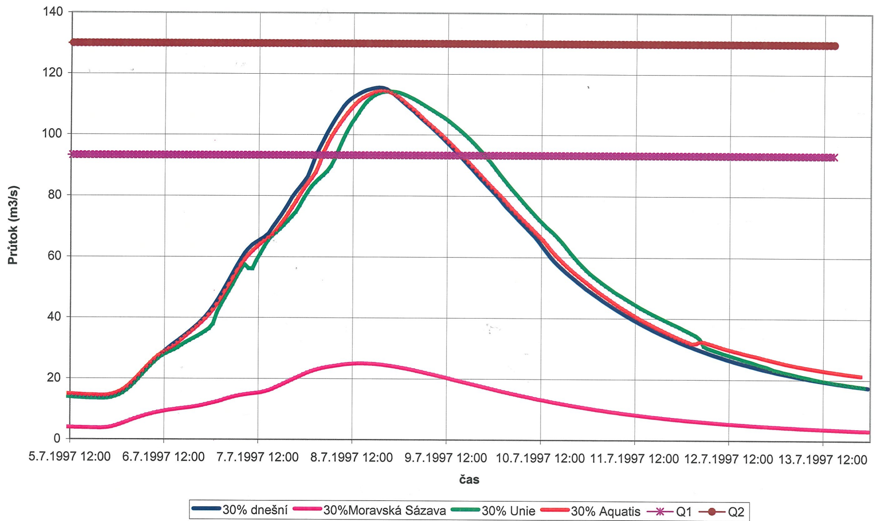
Povodeň v profilu pod Moravskou Sázavou vyvolaná 30% srážkových úhrnů povodně 1997
