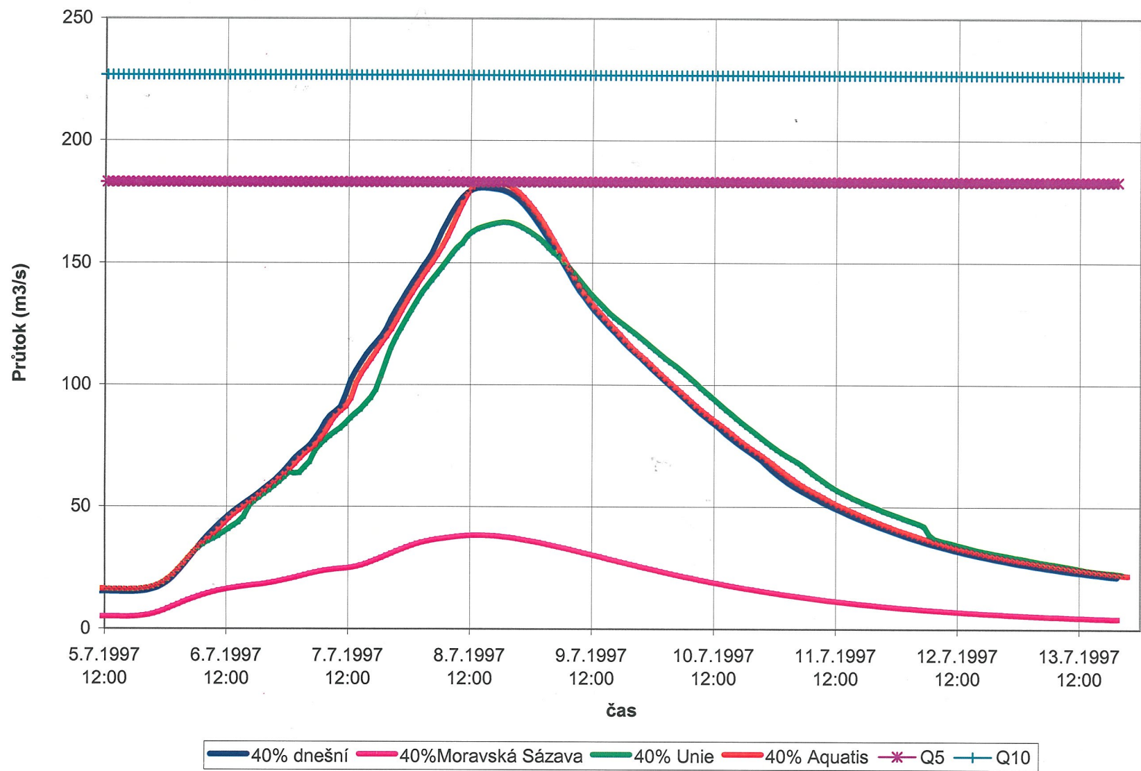
Povodeň v profilu pod Moravskou Sázavou vyvolaná 40% srážkových úhrnů povodně 1997
