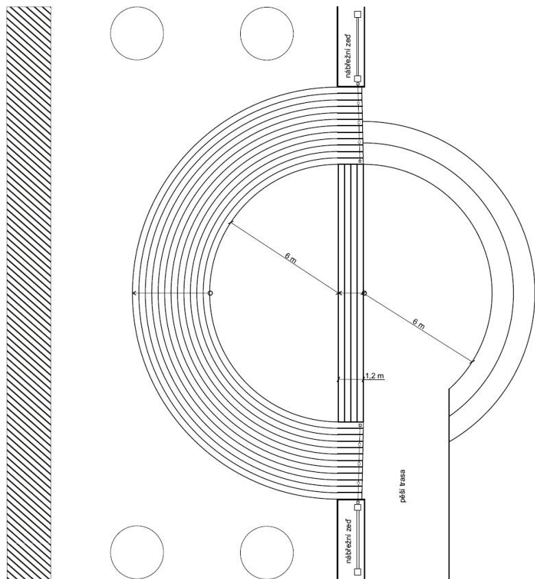
VSTUP A VÝSTUP NA NÁBŘEŽNÍ PĚŠÍ TRASU PŮDORYS - DETAIL
