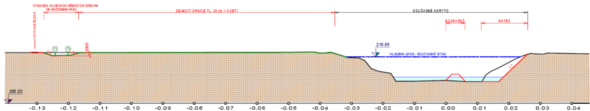
VZOROVÝ PŘÍČNÝ ŘEZ Č. 1
