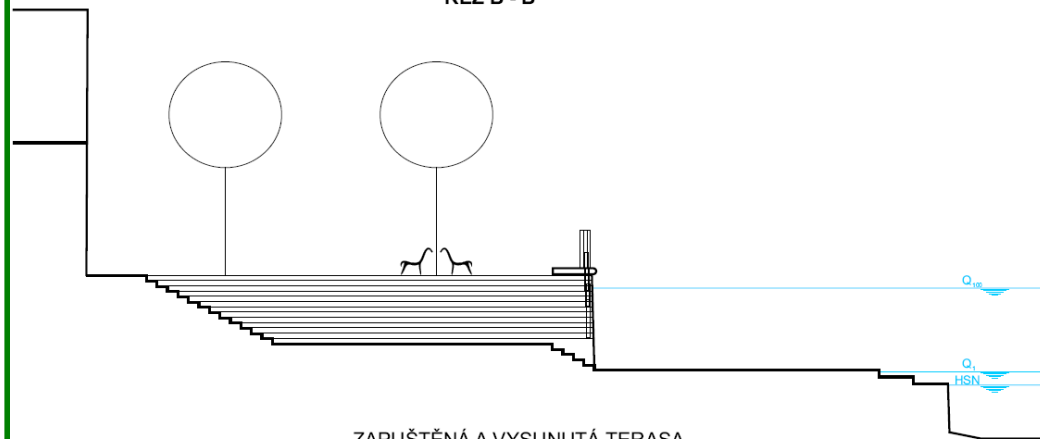
ZAPUŠTĚNÁ A VYSUNUTÁ TERASA
